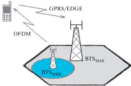
Рис. 8. Использование OFDM только на линии вниз
